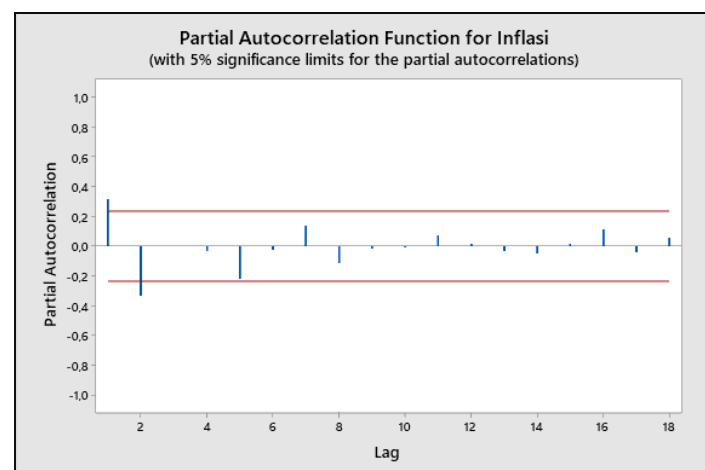
Gambar 4. Partial Autocorrelation Function (PACF) Inflasi Kota Padang
