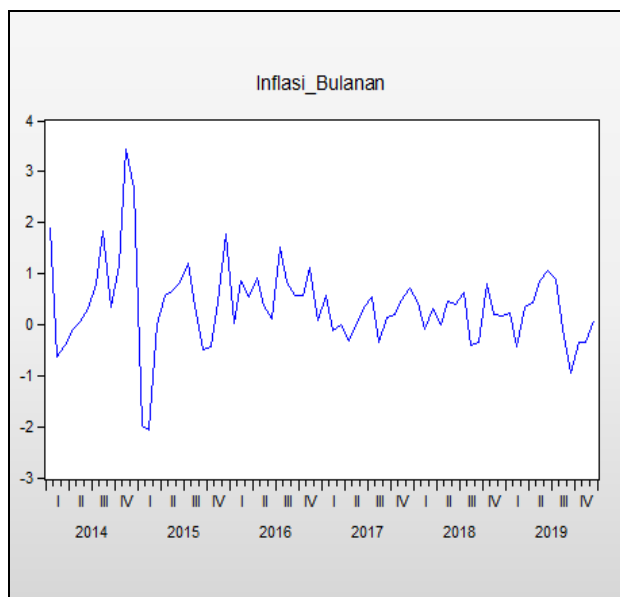
Gambar 1. Plot Data Inflasi Kota Padang Periode Januari 2014 – Desember 2019
