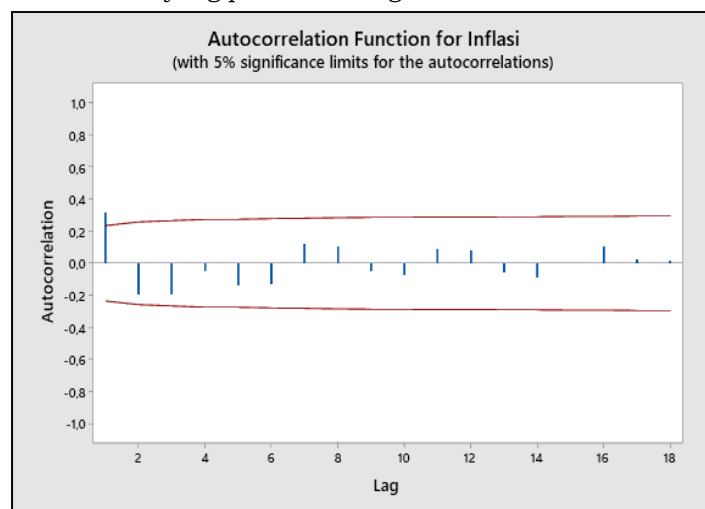
Gambar 3. Autocorrelation Function (ACF) Inflasi Kota Padang
