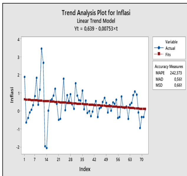
Gambar 2. Trend Analysis Inflasi Kota Padang
